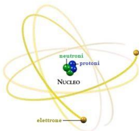
Fig. 4: modello atomico
